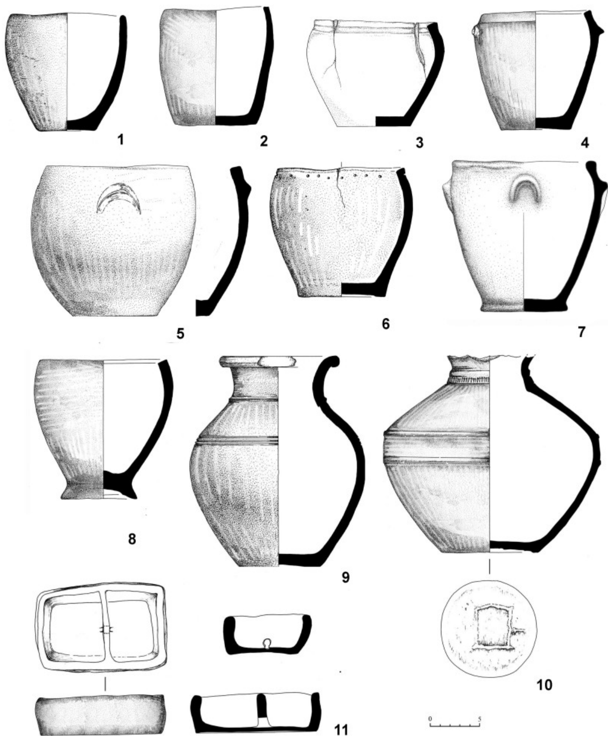
Рис. 2 Керамика. Могильник Ала-Тей 1
